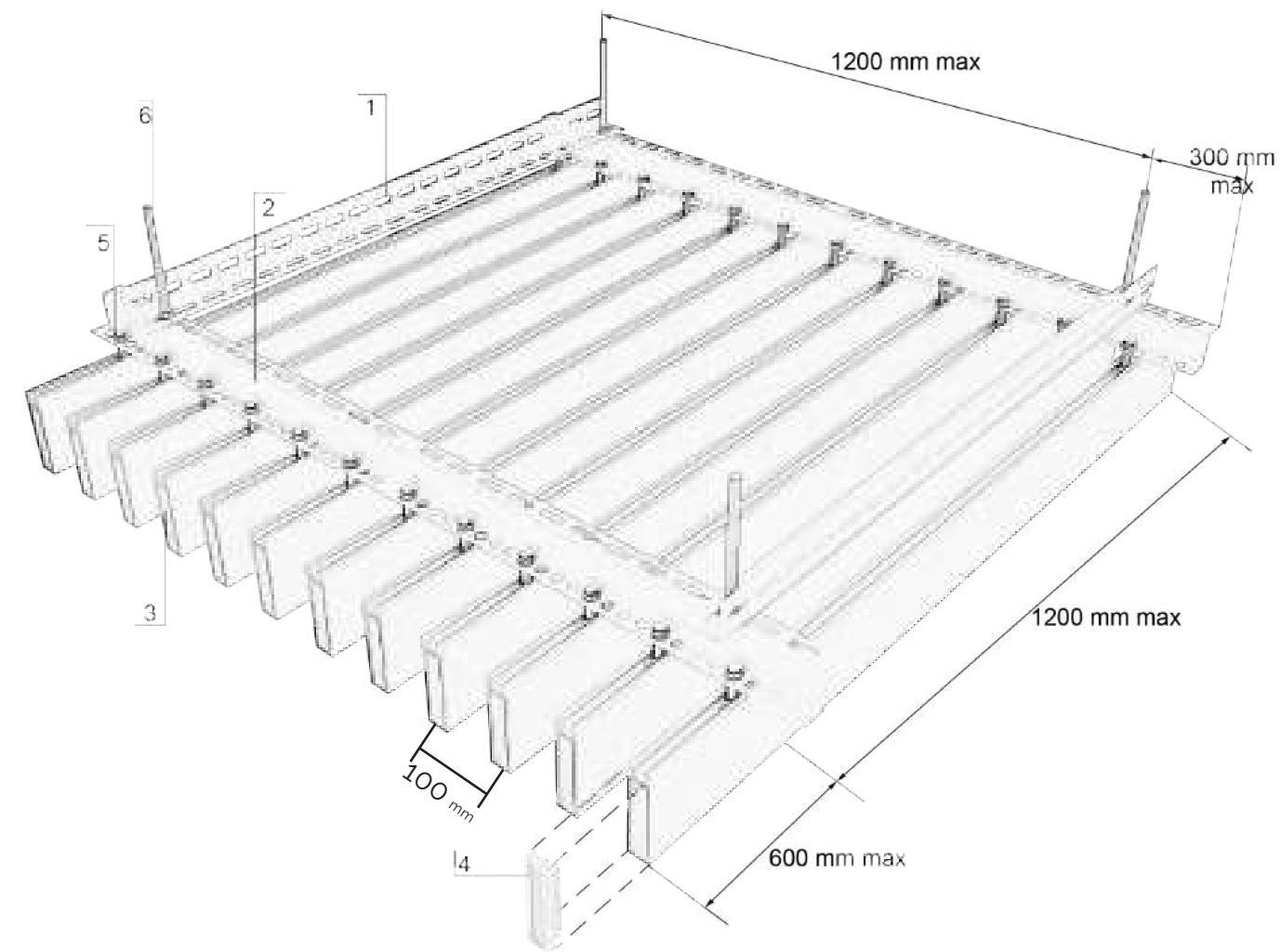
1- L Profil 2- Z Profil 3-Baffle 4- Cap 5- Bolt, Nut, Washer 6-Hanger Rod
