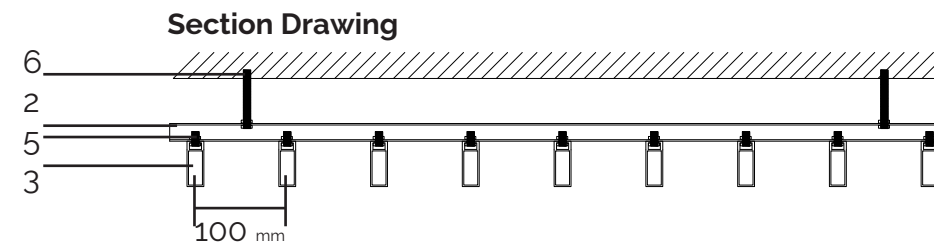
1- L Profil 2- Z Profil 3-Baffle 4- Cap 5- Bolt, Nut, Washer 6-Hanger Rod
